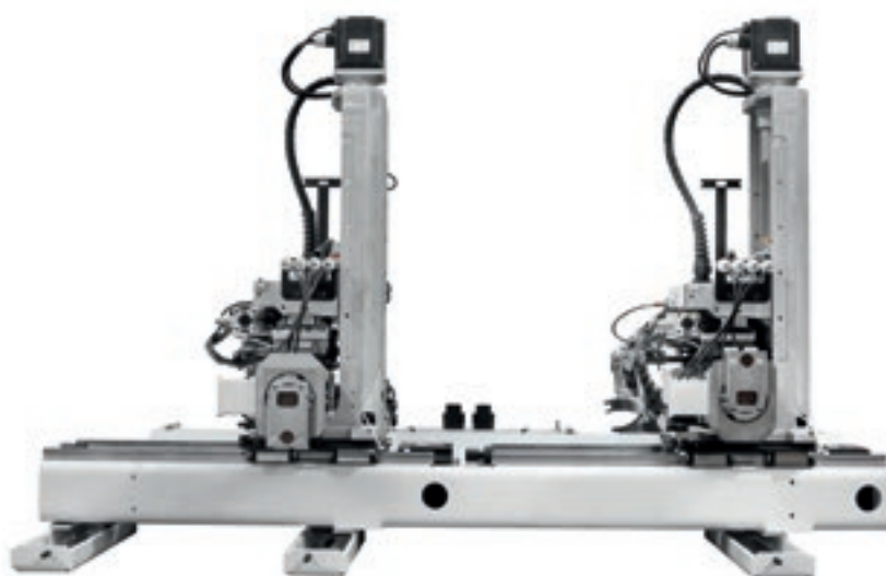
AR80 Закруглитель с 2 двигателями и приводом от бесколлекторного двигателя для высокоскоростной обработки и максимального качества и производительности.
